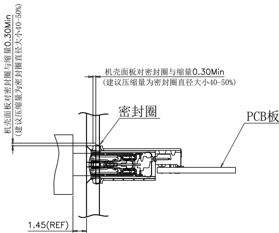
组装面板后公母头对插示意图
